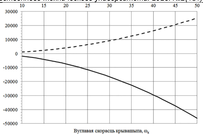
Рысунк 12 – Графік змянення тангенцыяльнай сілы \tilde{R}_{A_2}^t
