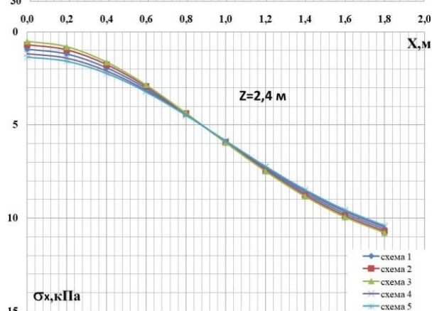
Рисунок 9 – Распределение горизонтальных напряжений \sigma_x в зависимости от расстояния от оси загрузки по глубине основания
