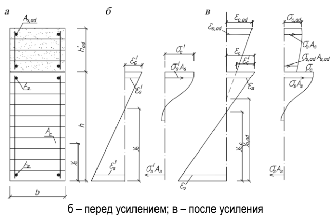
Рисунок 1 – Расчетное сечение изгибаемого железобетонного элемента, усиленного увеличением поперечного сечения в сжатой зоне (а) и распределение относительных деформаций и напряжений
