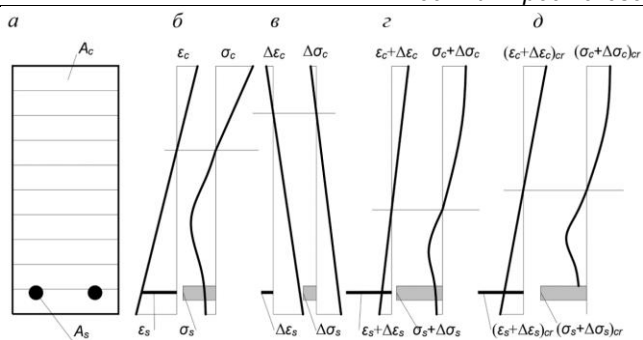
а) модель поперечного сечения изгибаемого элемента; б) относительные деформации и напряжения перед образованием трещины; в) дополнительные относительные деформации и напряжения; г) после приложения дополнительной относительной деформации (напряжения) от взаимного сдвига бетона и арматуры; д) после образования трещины
