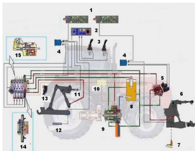
Рисунок 1 – Функциональная схема электрогидравлической системы управления рабочими органами трактора «Беларус МТЗ-3022»
